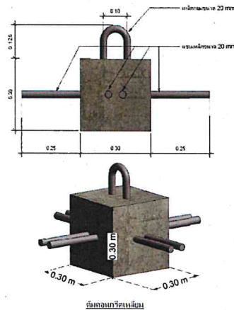
ลักษณะฐานทุ่นสำหรับทำขี้งเชือก
