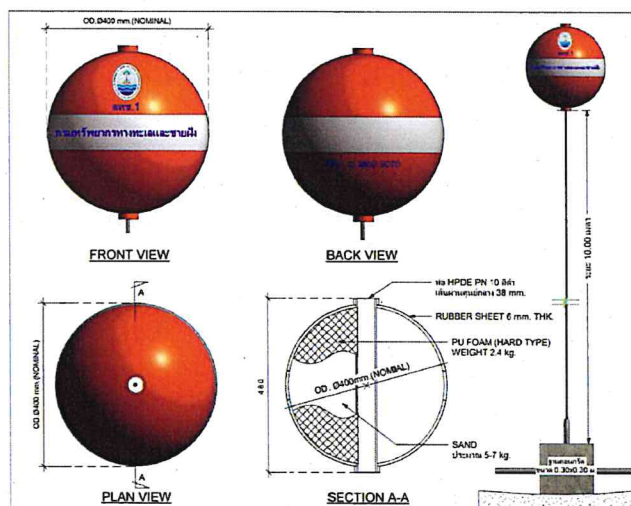
ลักษณะทุ่นทำซั้งเชือก
