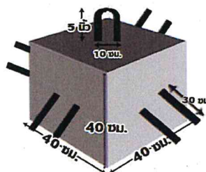
ลักษณะฐานทุ่นแสดงแนวเขต
