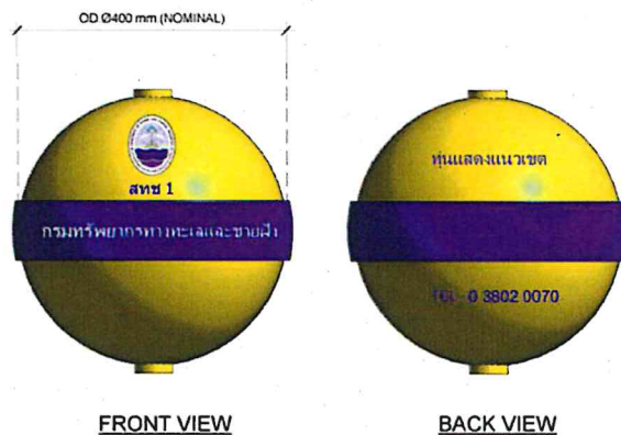
รูปแบบลักษณะทุ่นแสดงแนวเขต
