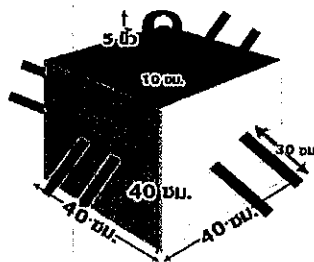
ลักษณะฐานทุ่นแนวเขตปะการังเทียม
