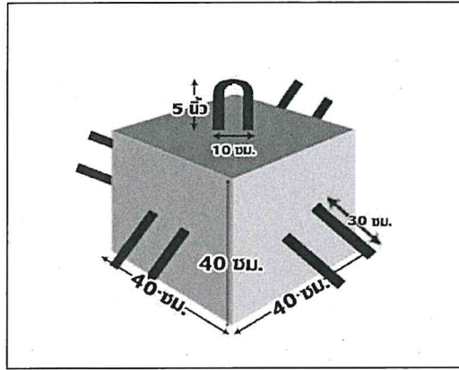
ลักษณะฐานท่อนแนวเขตดักขยะ
