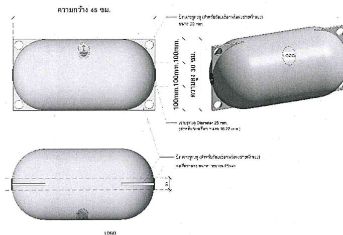
ลักษณะหุ่นกันขยะ
