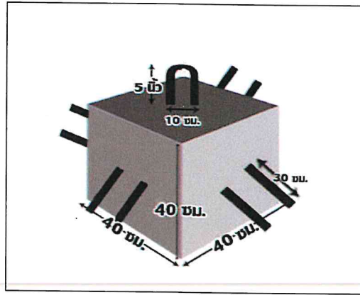
ลักษณะฐานหุ่นผูกเรือ
