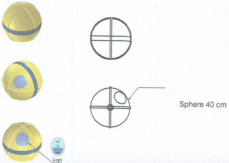
ลักษณะทุ่นกำหนดเขตพื้นที่อนุรักษ์
