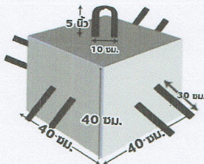
ลักษณะฐานทุ่นกำหนดเขตพื้นที่อนุรักษ์
