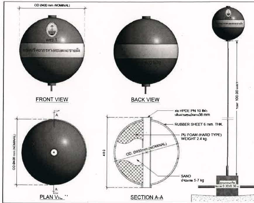
ลักษณะทุ่นทำขังเชือก
