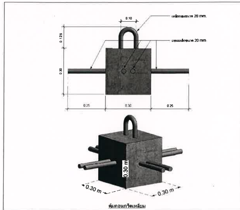
ลักษณะฐานหุ่นทำขังเชือก
